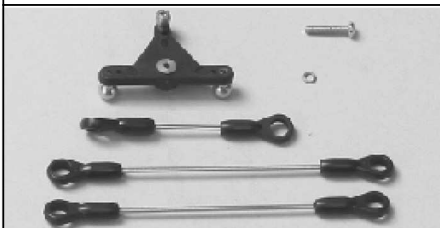
50 050 8374 Rocker components set Anlenk-/ Gestängeset
