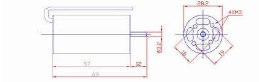
Abmessungen / Dimension Ø 28,2x57 mm
