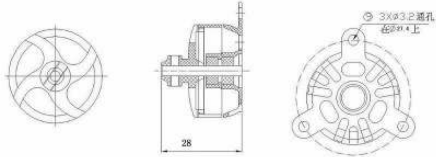
Abmessungen / Dimension Ø 27.4X24 mm
